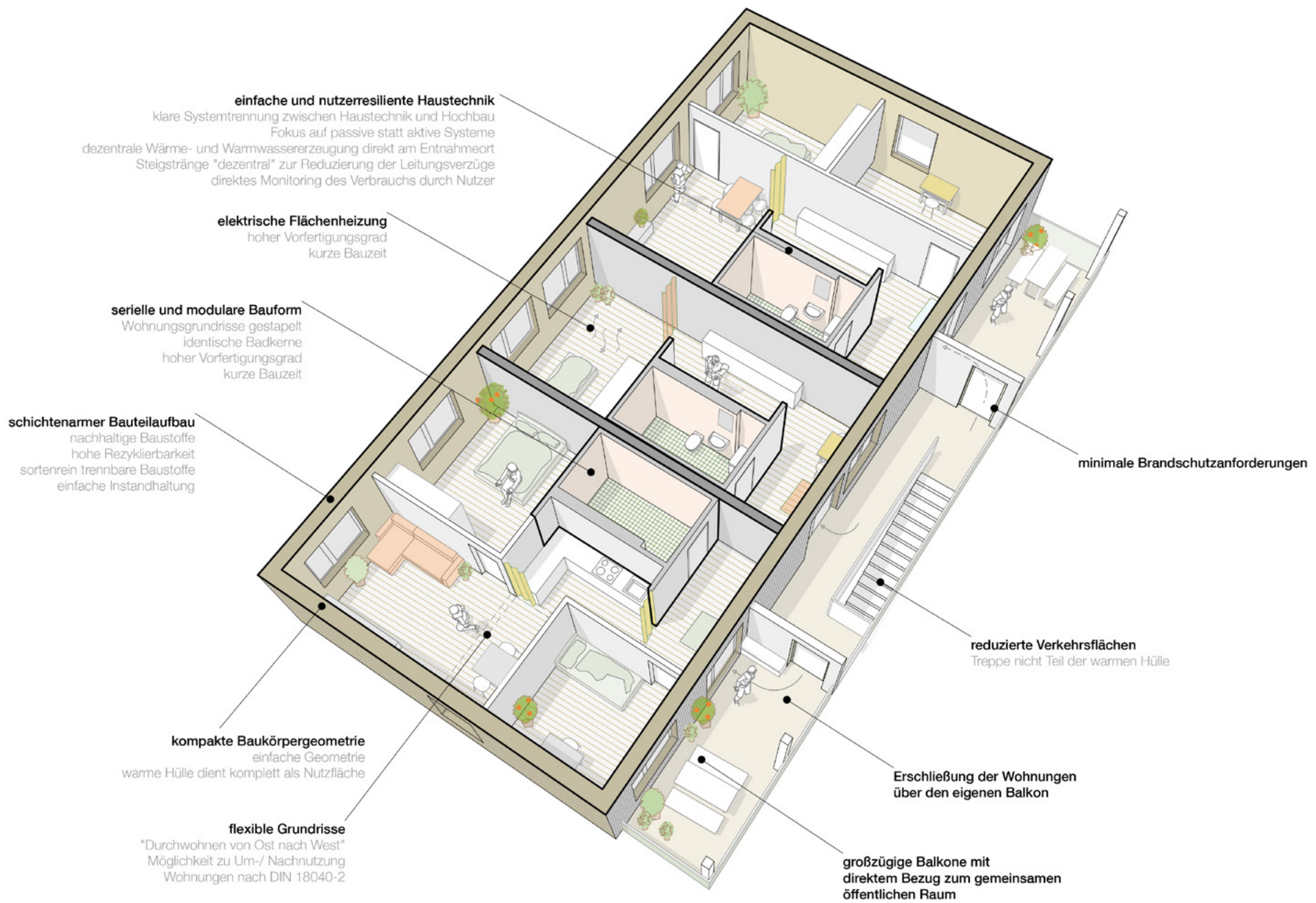
Weitere Kennzeichen des Konzepts für sechs Wohnhäuser in Augsburg-Haunstetten, dargestellt anhand des Grundrisses eines Regelgeschosses. Plan: hey! architektur / IGEWO
